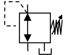
Basınç ayar valfi (3 yollu)
