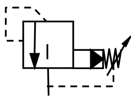
Pilotlu Basınç sınırlama valfi
