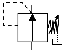
Basınç ayar valfi (2 yollu)
