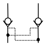
Çift pilotlu çek valf
