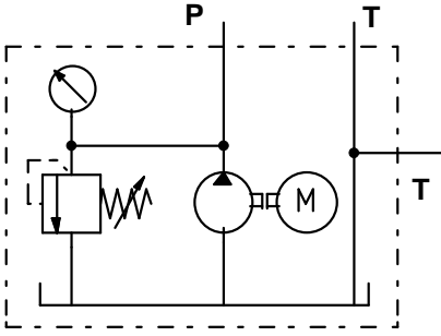
Hidrolik güç ünitesi
