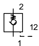
İkazlı çek valf
